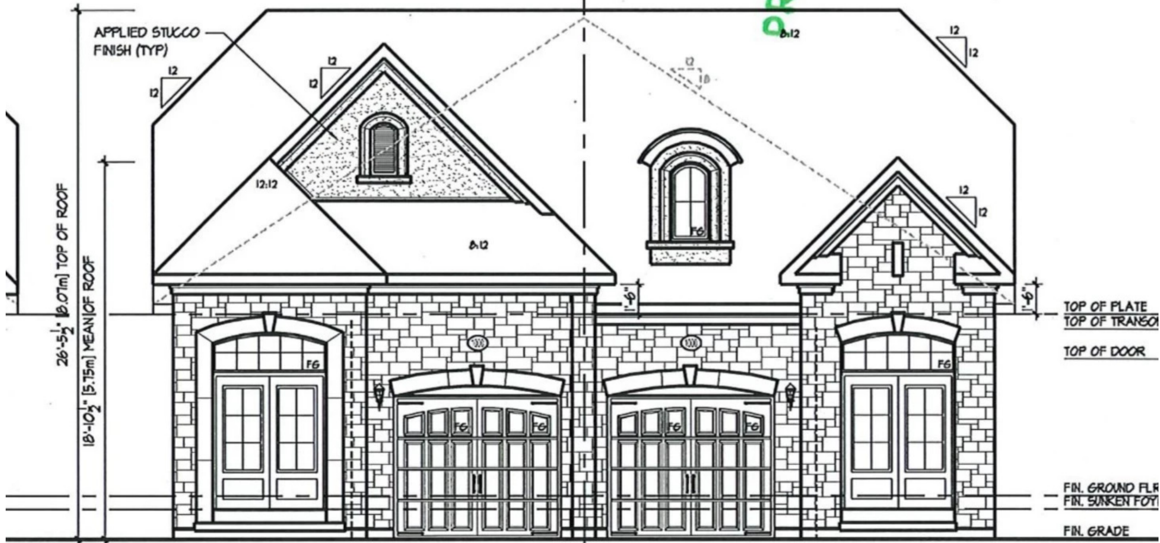
FRONT ELEVATION 'B-1'
